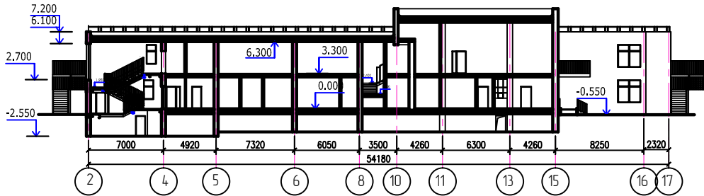
Разрез 2-2
