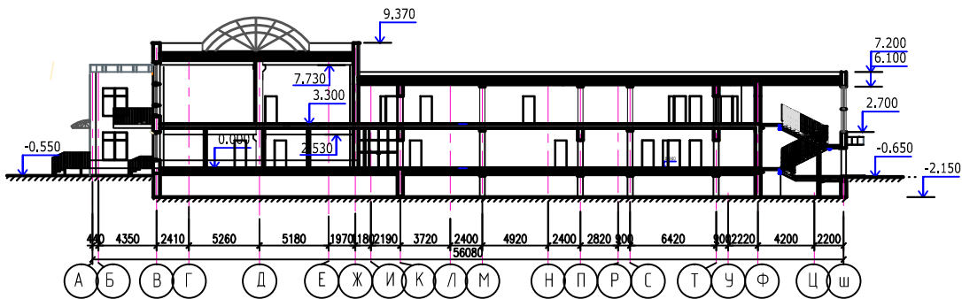
Разрез 1-1
